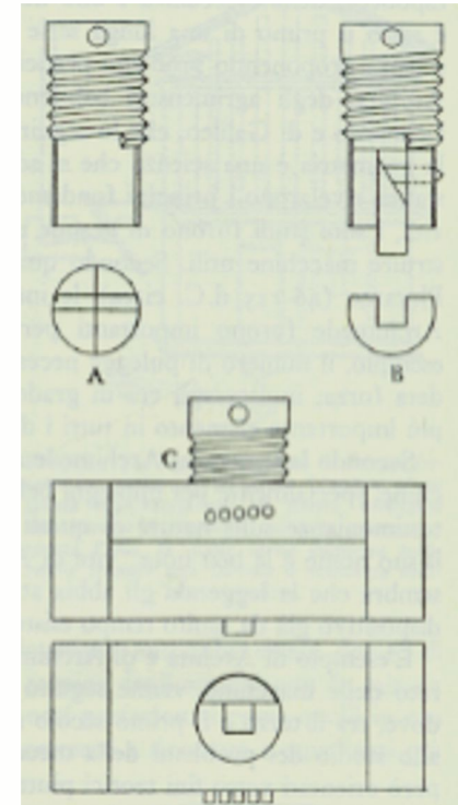
FIGURA 572—Ricostruzione della filettatrice di Erone. (a) Pianta e alzata del manico della filettatura. Esso ha un foro per il manico all'estremità superiore e un piolo a quello inferiore. (b, sopra) Un'asola è stata eseguita nel piolo e in essa è stata fissata una fresa di ferro — notare il bordo di taglio obliquo — destinata a produrre la filettatura della madrevite segnando una linea continua. (b, sotto) L'estremità del piolo vista di sotto. (c, sopra) La vite con il piolo così preparato è inserita nel foro di una tavola. Cinque piccoli pioli sul lato della tavola formano una sorta di filettatura provvisoria per guidare la fresa. La madrevite è tagliata nella seconda tavola, anch'essa attraversata da un foro. (c, sotto) Pianta della filettatrice in azione. Notare che un terzo del cono segato nell'eseguire l'asola è stato sostituito.
