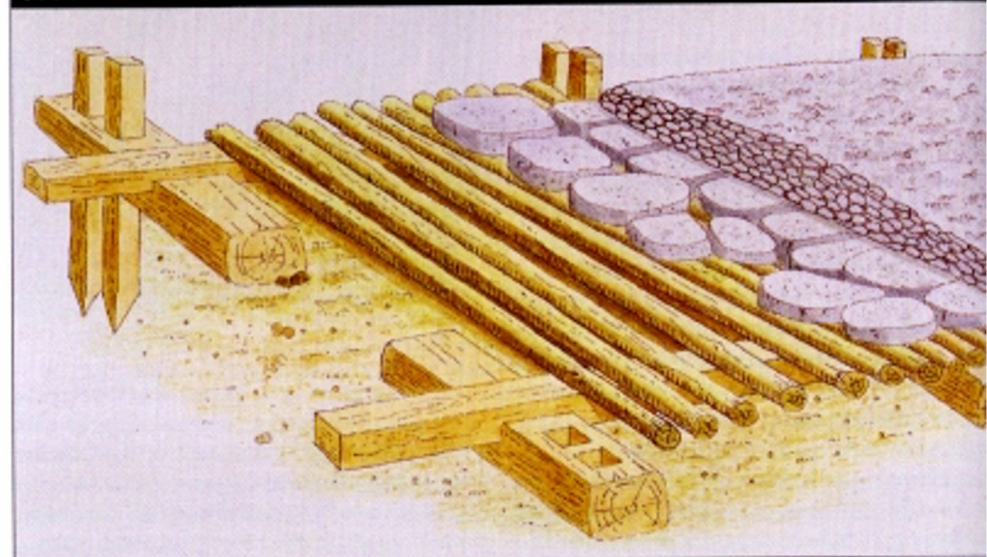
Sezione di una strada romana
