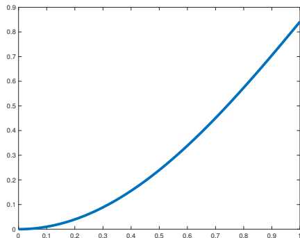
Figura: Grafico della funzione f(x) = x \cdot \sin(x) , nell'intervallo [0, 1] .
