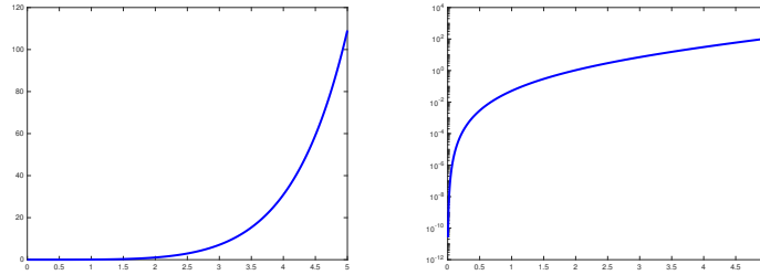
Figura 4: Differenza tra plot e semilogy nel rappresentare i grafici unendo mediante un segmento le coppie (x_k, |f(x_k) - p(x_k)|) per t = 1, \dots, 1000 .
