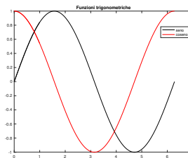
Figura 7: Grafico di \sin(x) , \cos(x) in [0, 2\pi] , con titolo e legenda.
