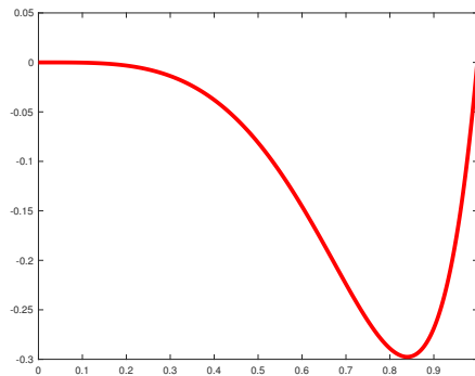
Figura 2: Grafico della funzione f(x) = \exp(x) \cdot \sinh(x) \cdot x^2 \cdot \tan(x) \cdot \log(x + 0.001) , nell'intervallo [0, 1] .
