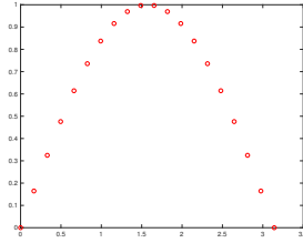
Figura 5: Grafico delle coordinate (x_k, \sin(x_k)) , per x_k = 0 + (k - 1)\pi/19 , k = 1, \dots, 20 .
