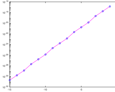
Figura 6: Grafico richiesto dall'esercizio.
