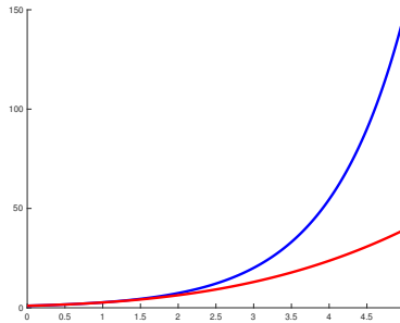
Figura 3: Grafico della funzione f(x) = \exp(x) (in blu), p(x) = 1 + x + \frac{x^2}{2} + \frac{x^3}{6} (in rosso), nell'intervallo [0, 5] .
