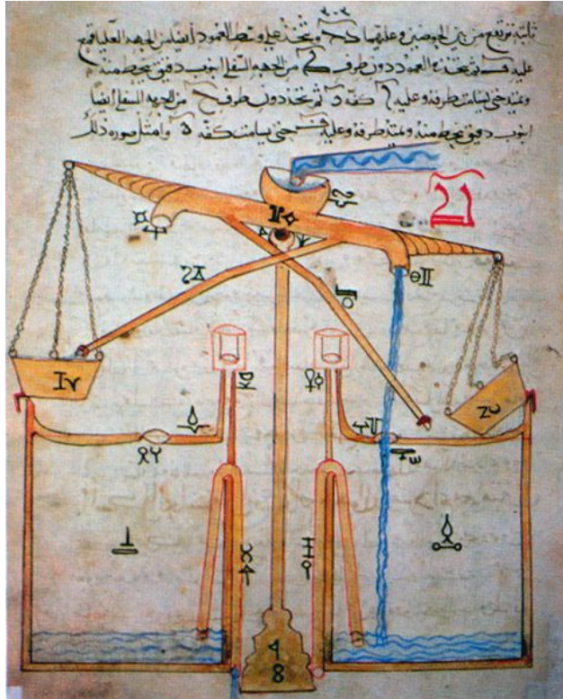
Macchina a bilanciere per sollevare l'acqua
