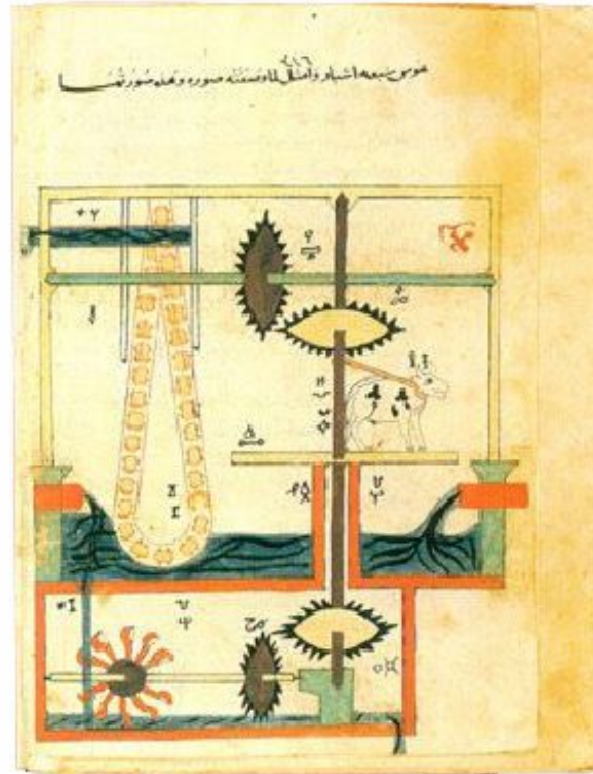
Macchina con noria per sollevare l'acqua
