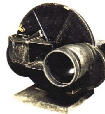
第1図 テレビジョン電話装置 昭和10年 (本体製造昭和8年)
